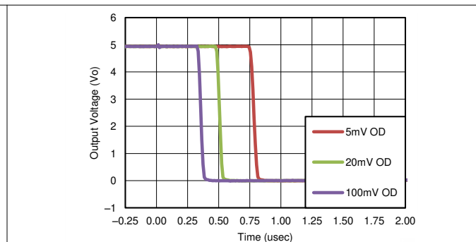
图 8-3. 各种过驱的响应时间 (负转换)
