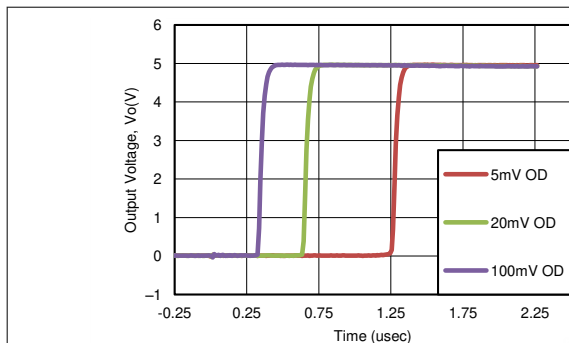
图 8-2. 各种过驱的响应时间 (正转换)
