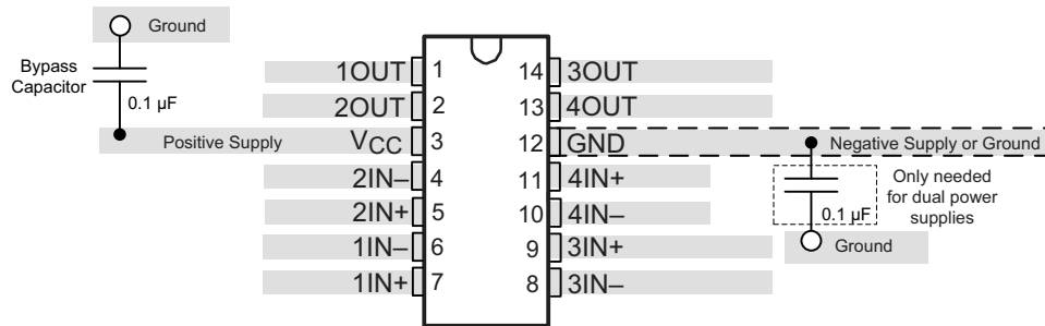
图 11-1. LMx39 Layout Example
